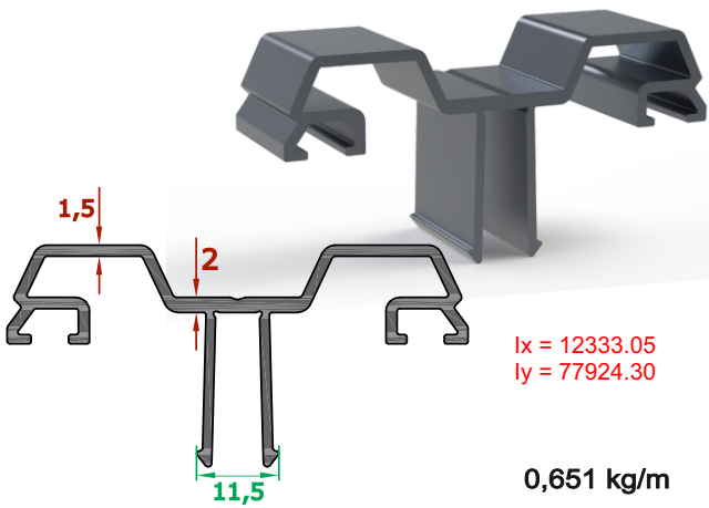
Cam Alt Baskı Profili (Cam Kapak)
