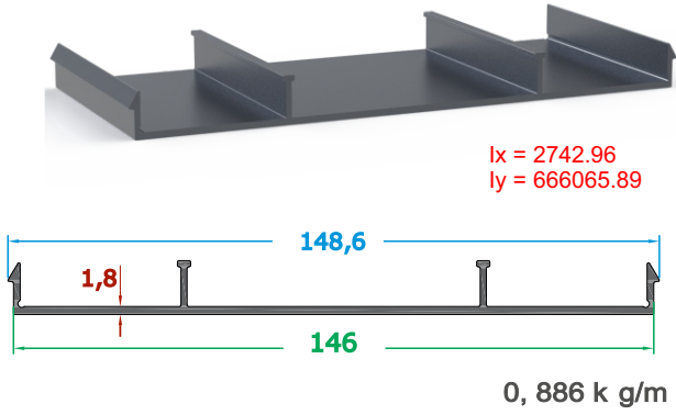
Oluk Alt Kapak Profili
