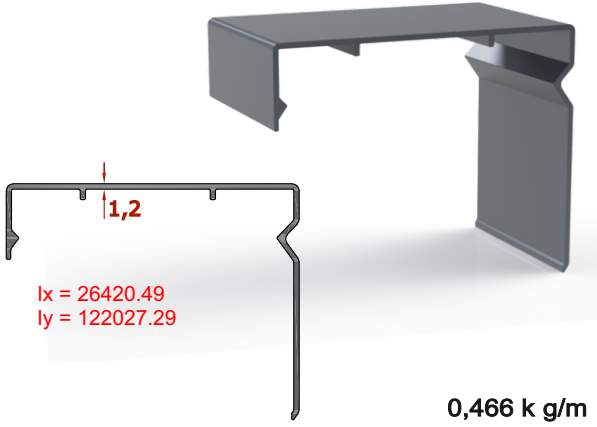
Üst Yan Kapak Profili (Yan Kapak)
