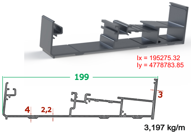
Duvar Tutucu Profili (Ara Tayıcı)
