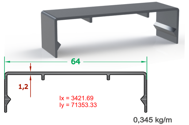
Üst Kapak Profili
