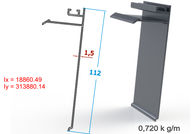
Oluk ve Arka Taşıyıcı Kapak Profili
