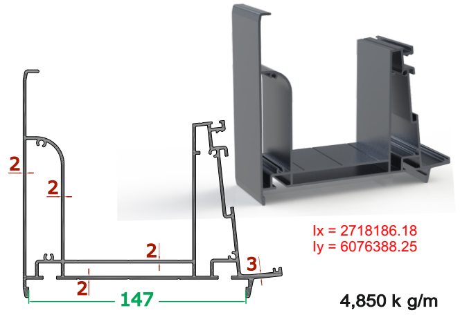
Düz Oluk Profili
